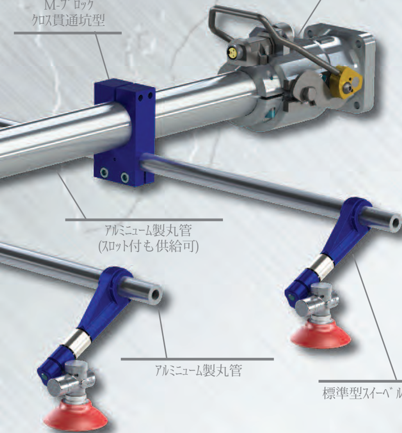
60mm/2.5" クイック脱着、電気接続付
