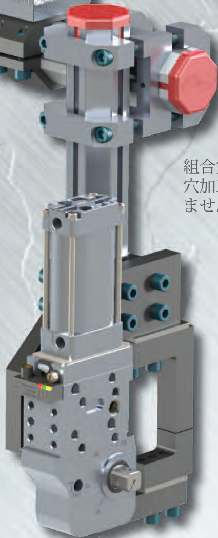
82M シリーズ パワークランプ
