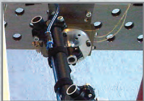
Accelerate® tooling装着の標準回転式チップ
